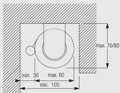
4803 Кронштейн (58 мм)
